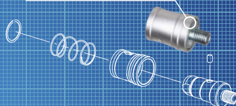
Переходник M18 – M16 система "click-clack"
